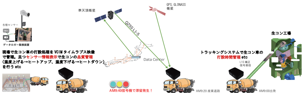
コンクリート打設管理イメージ
